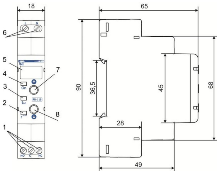
Рисунок 1 – Органы управления, габаритные и установочные размеры RN-118/RN-119
